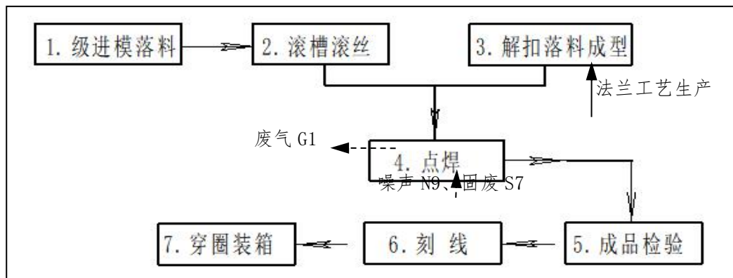
图4-4 项目桶塞环生产工艺流程图示意图
