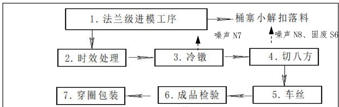
图4-3 项目法兰生产工艺流程示意图
