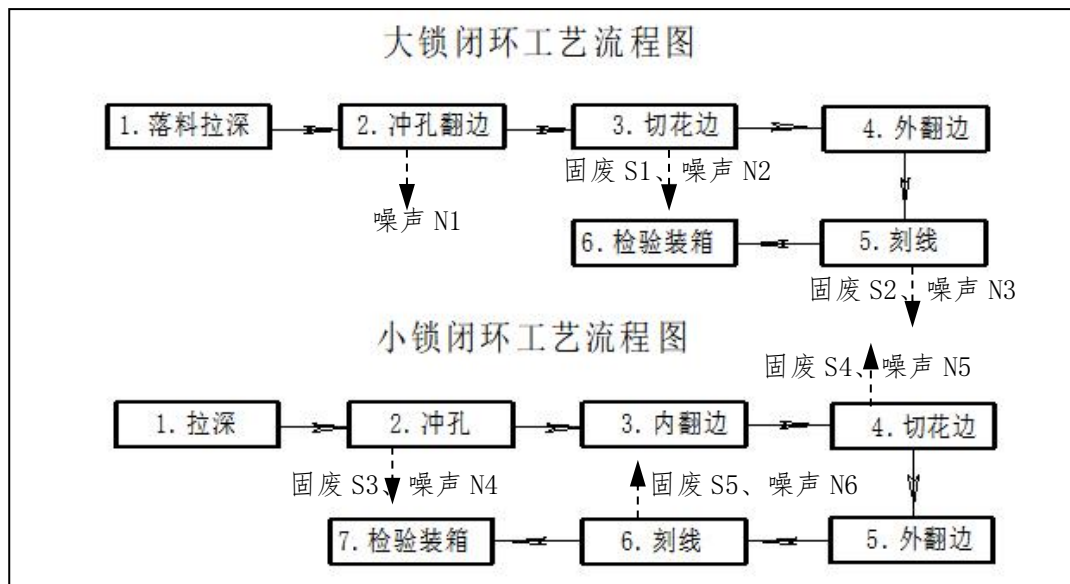
图4-2 项目锁闭环生产工艺流程示意图
