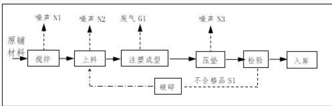
图 4-5 项目塑料瓶生产线工艺流程及产污环节简图
