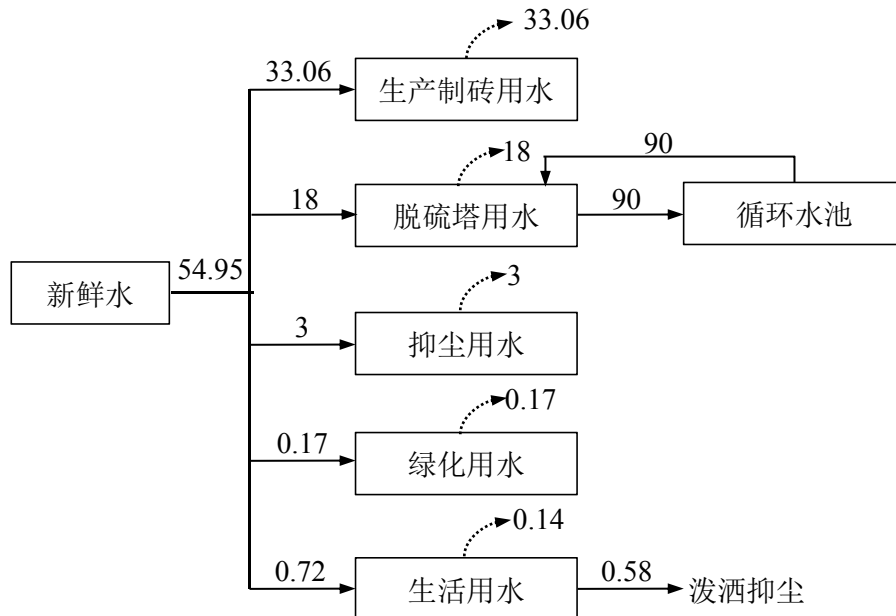
图 2.5-7 项目给排水平衡示意图 m 3 /d
