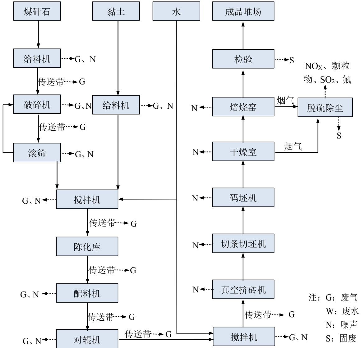
图 2.5-4 项目生产工艺流程及排污节点图
