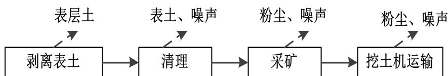
图 2.5-3 粘土开采工艺流程及产污环节示意图
