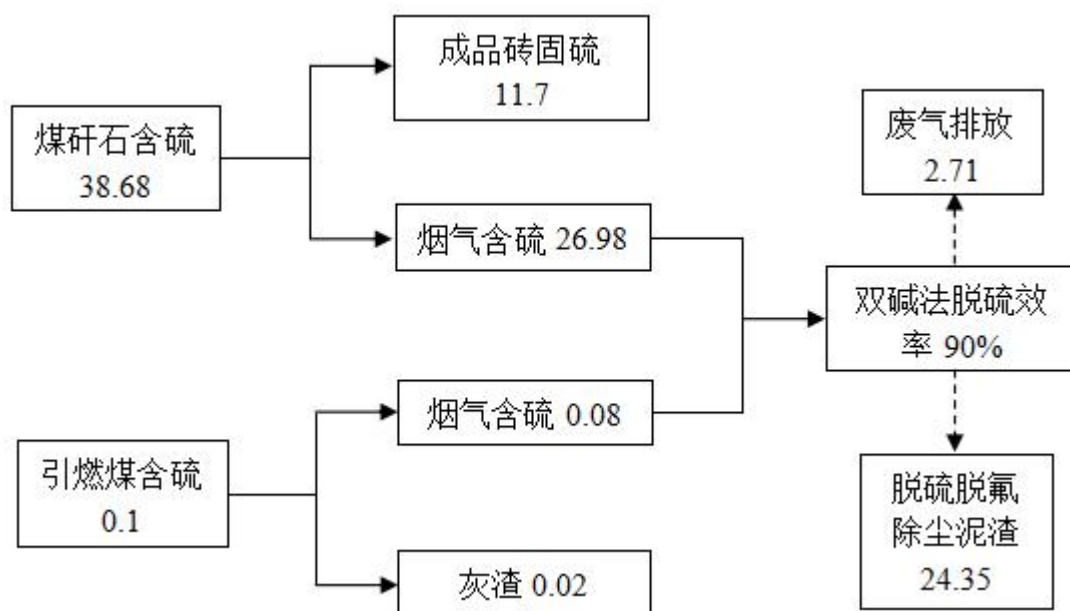
图 2.5-5 硫平衡图 单位: t/a
